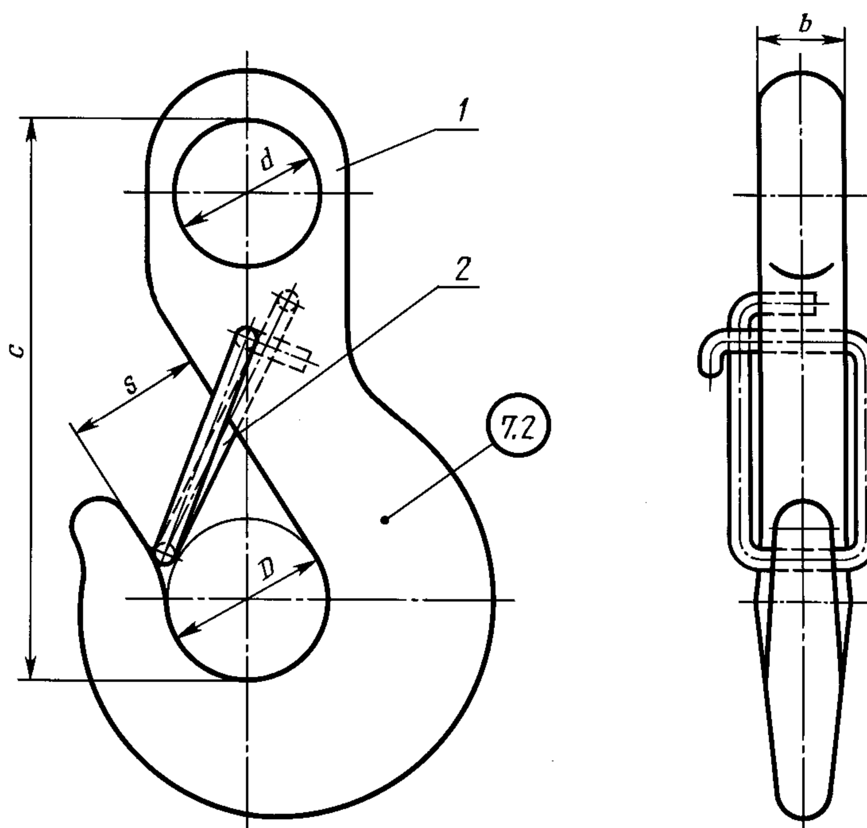
1 — крюк; 2 — замок
