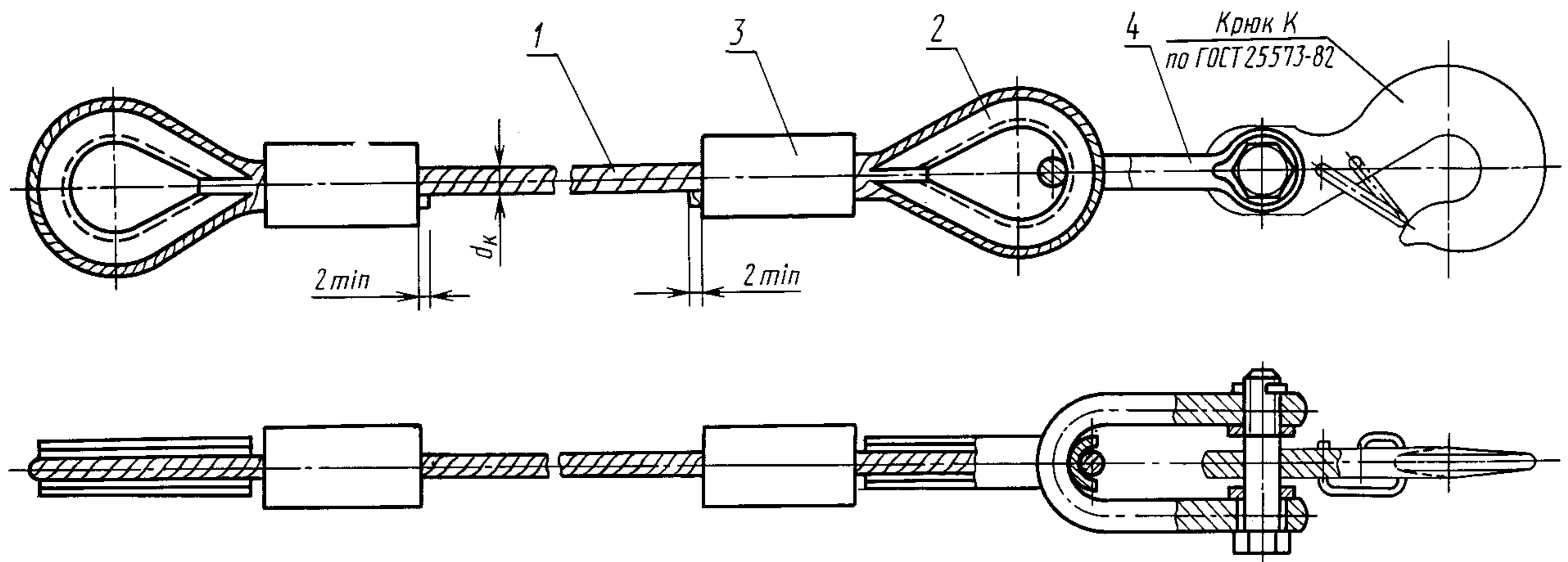
Канатная ветвь с переходным звеном
