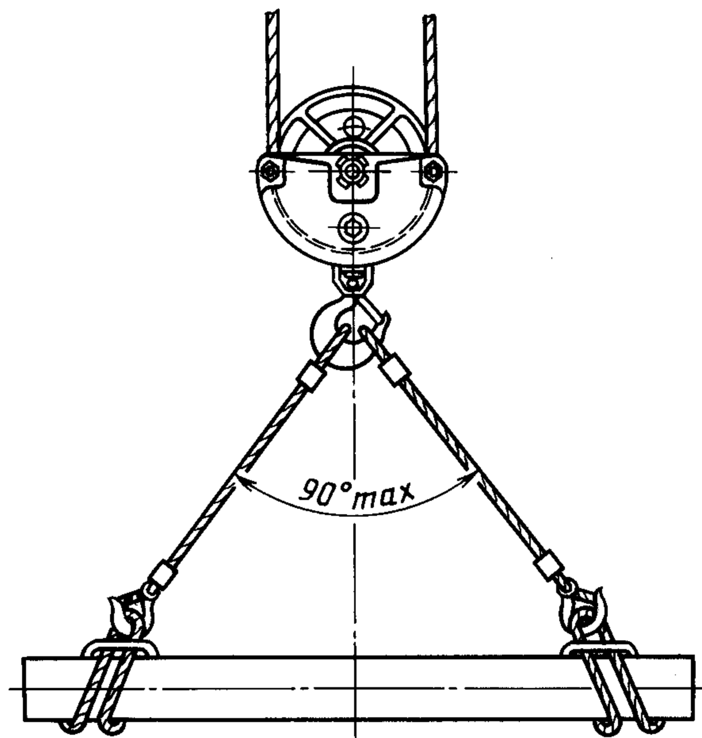
Схема строповки грузов стропами СКП2
