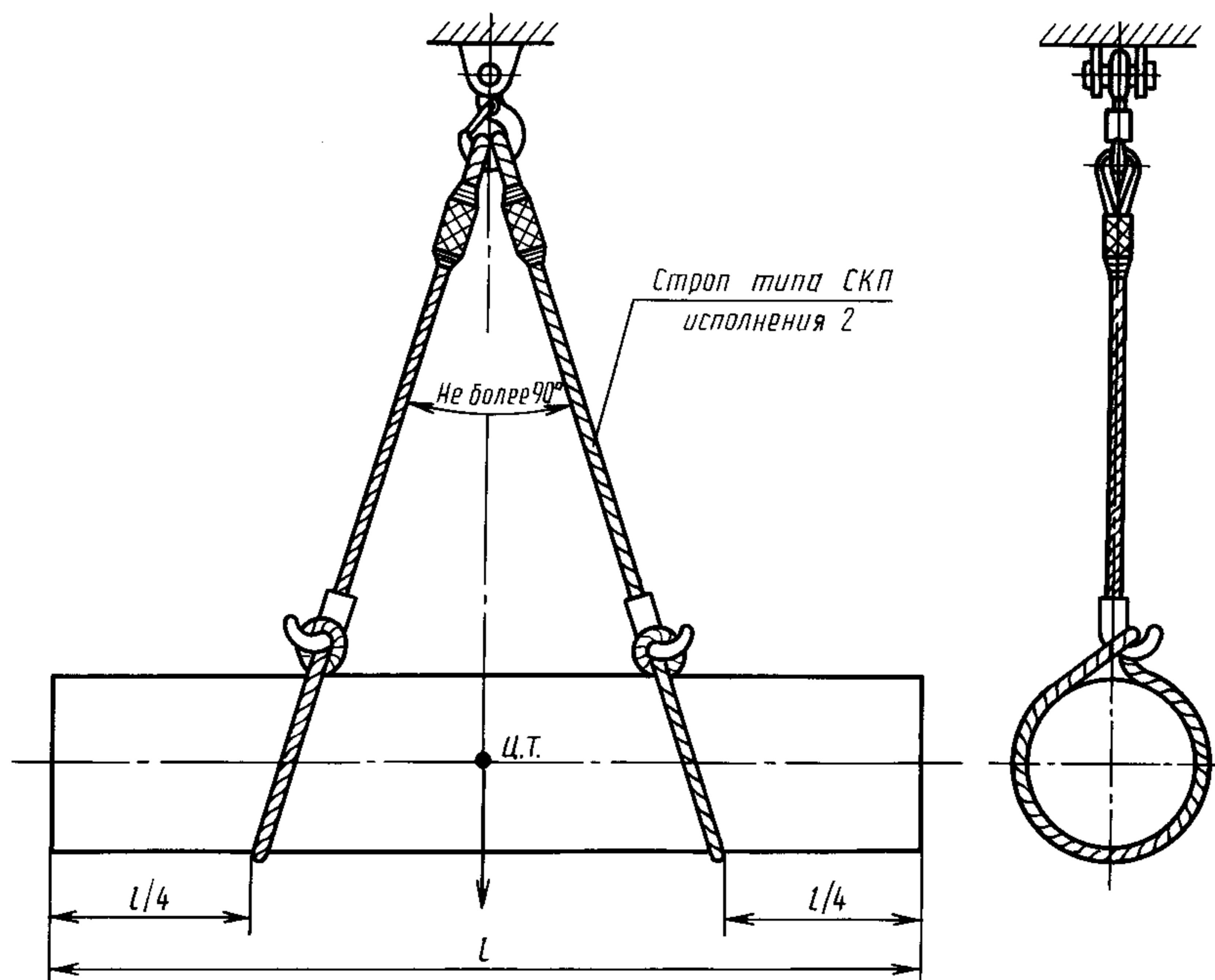
Схема строповки грузов стропами СКП2
